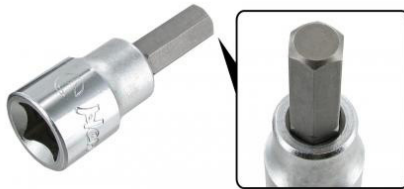
Douille tournevis à 6 pans douille 8 mm pour cliquet 3/8 pouce pour tous les modèles à cardan, pour le train avant du Combi T3 Syncro
