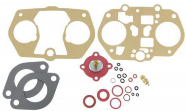
Kit de rénovation/révision pour carburateur Dellorto DRLA 36, DRLA 40, EMPI D 36mm, D 40mm
